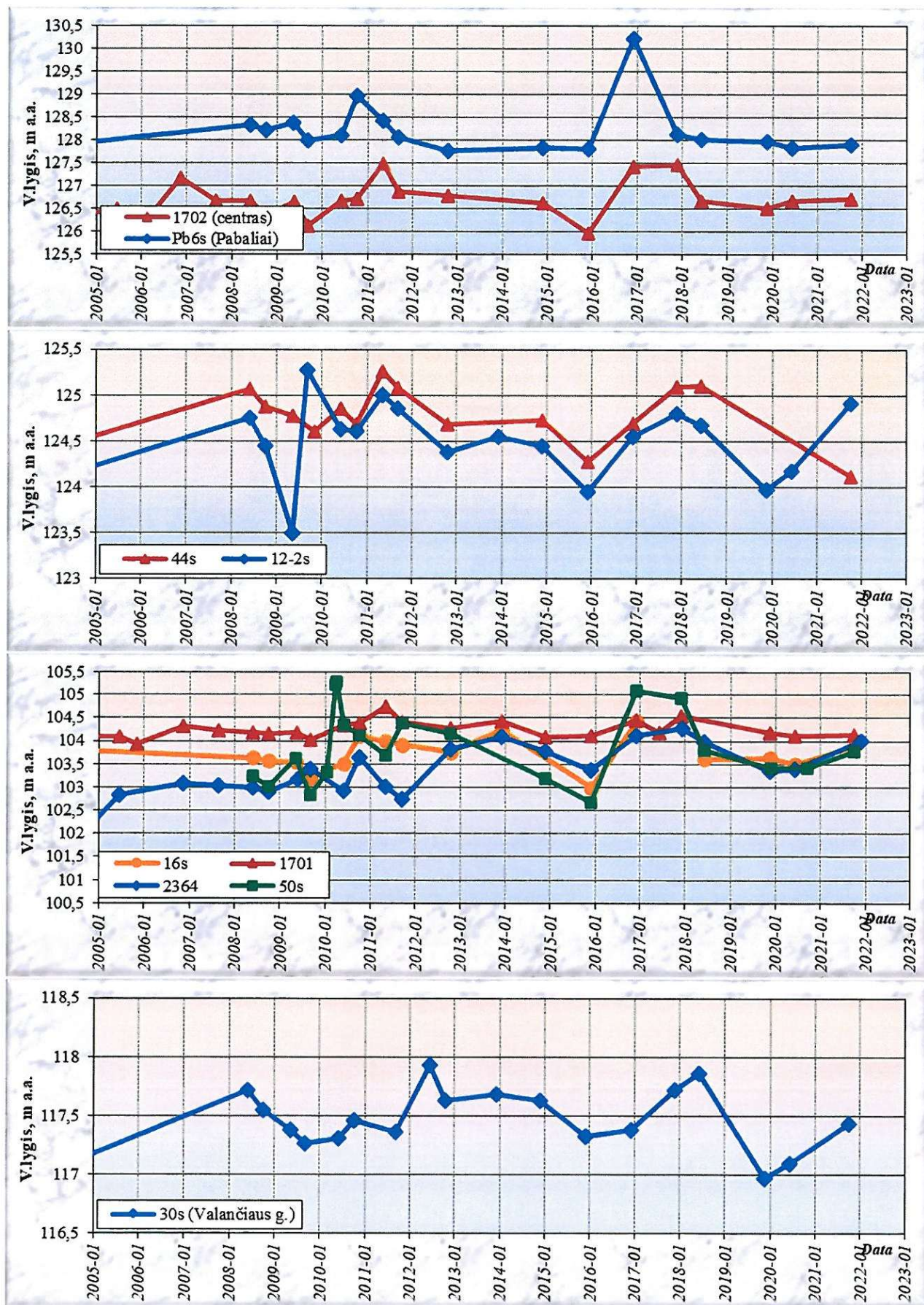
4 pav. Gruntinio vandens lygių kaitos grafikai (2005–2021 m.)
