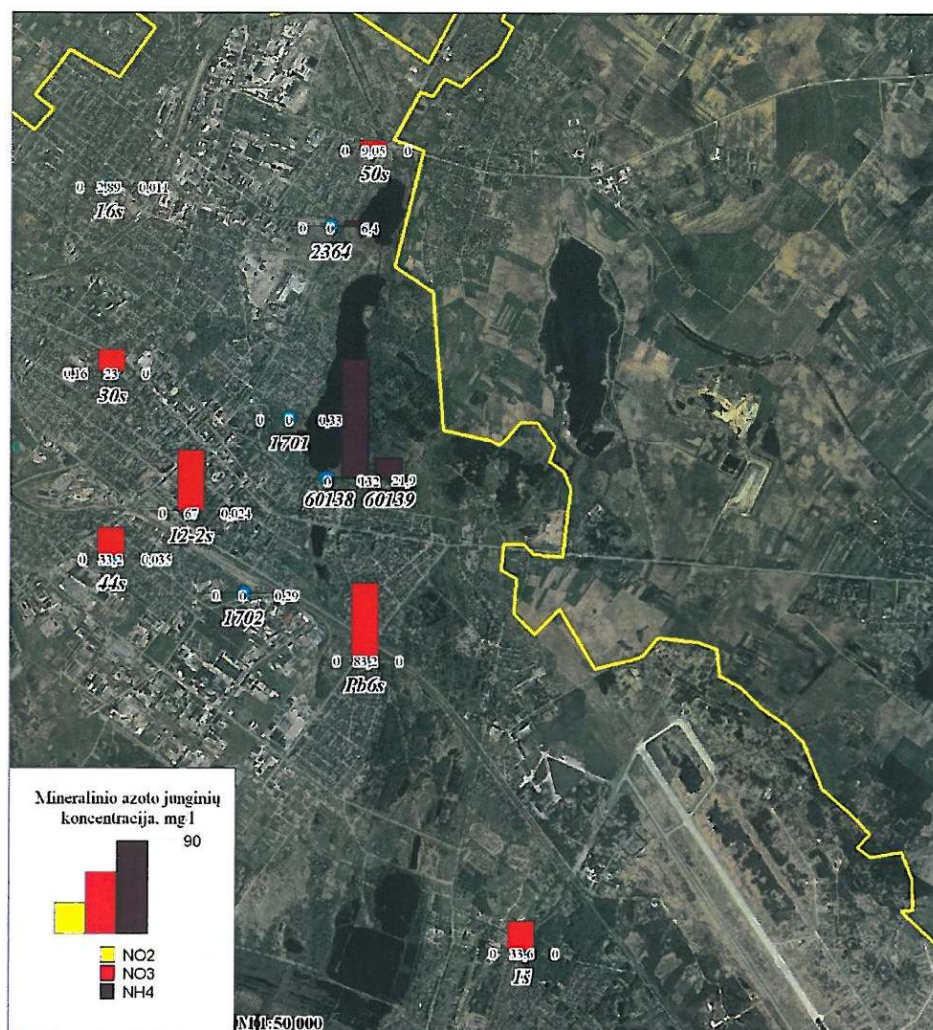
8 pav. Mineralinio azoto koncentracija gruntiniame vandenyje (2021 m.)
