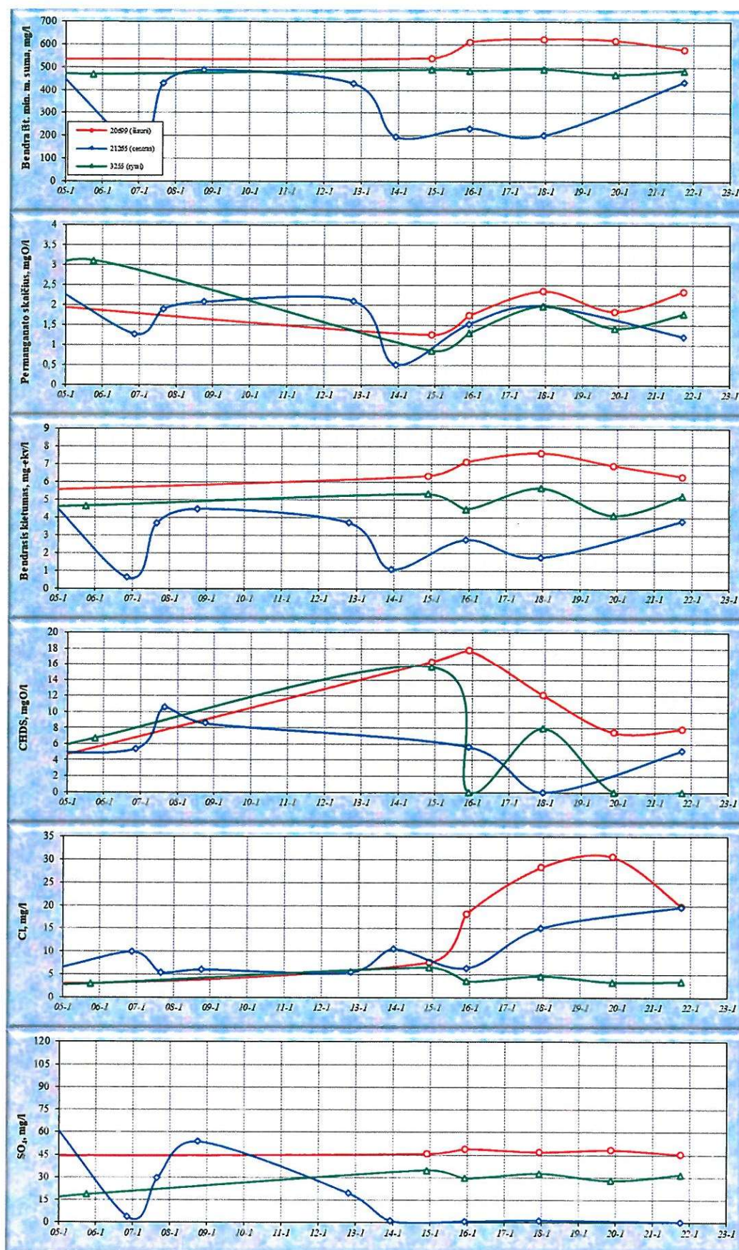
12 pav. Permo sluoksnio požeminio vandens cheminės sudėties rodiklių kaita (2005–2021 m.)
