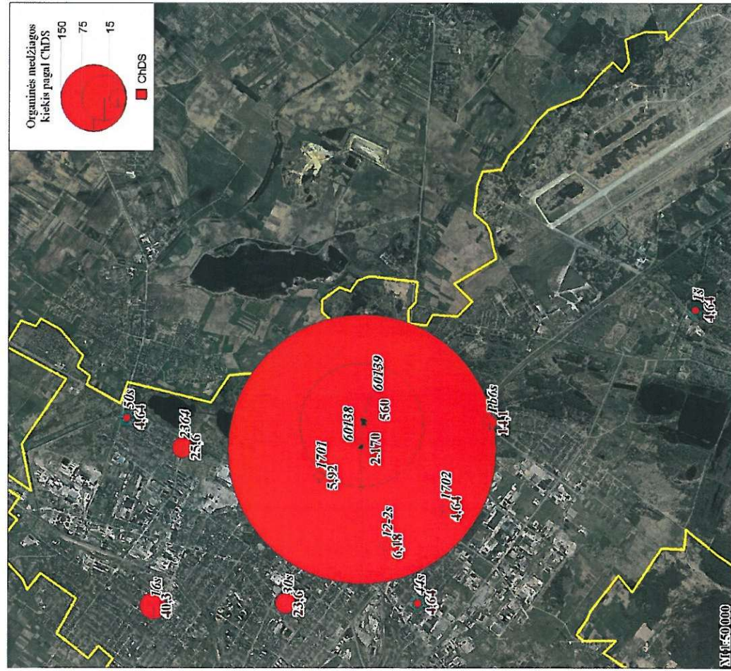
6 pav. ChDS vertės gruntuose vandenyje (2021 m.)
