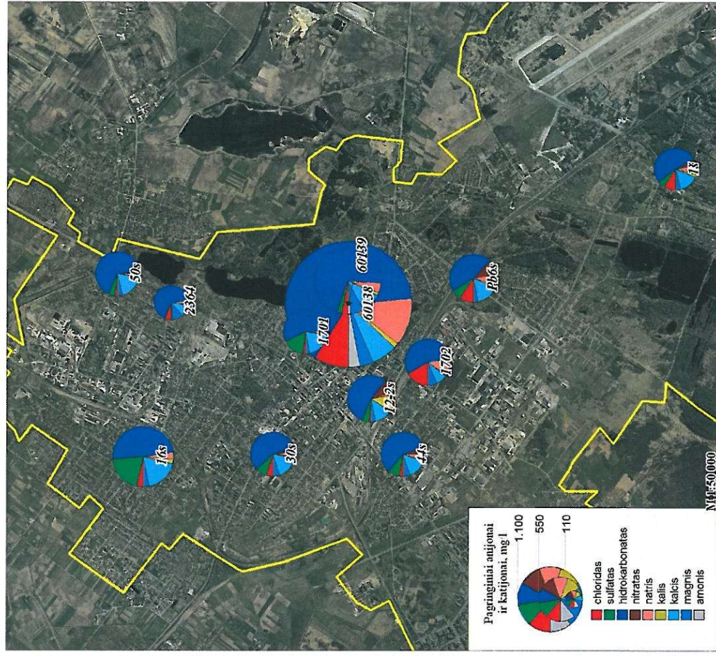
7 pav. Gruntinio vandens cheminė sudėtis (2021 m.)
